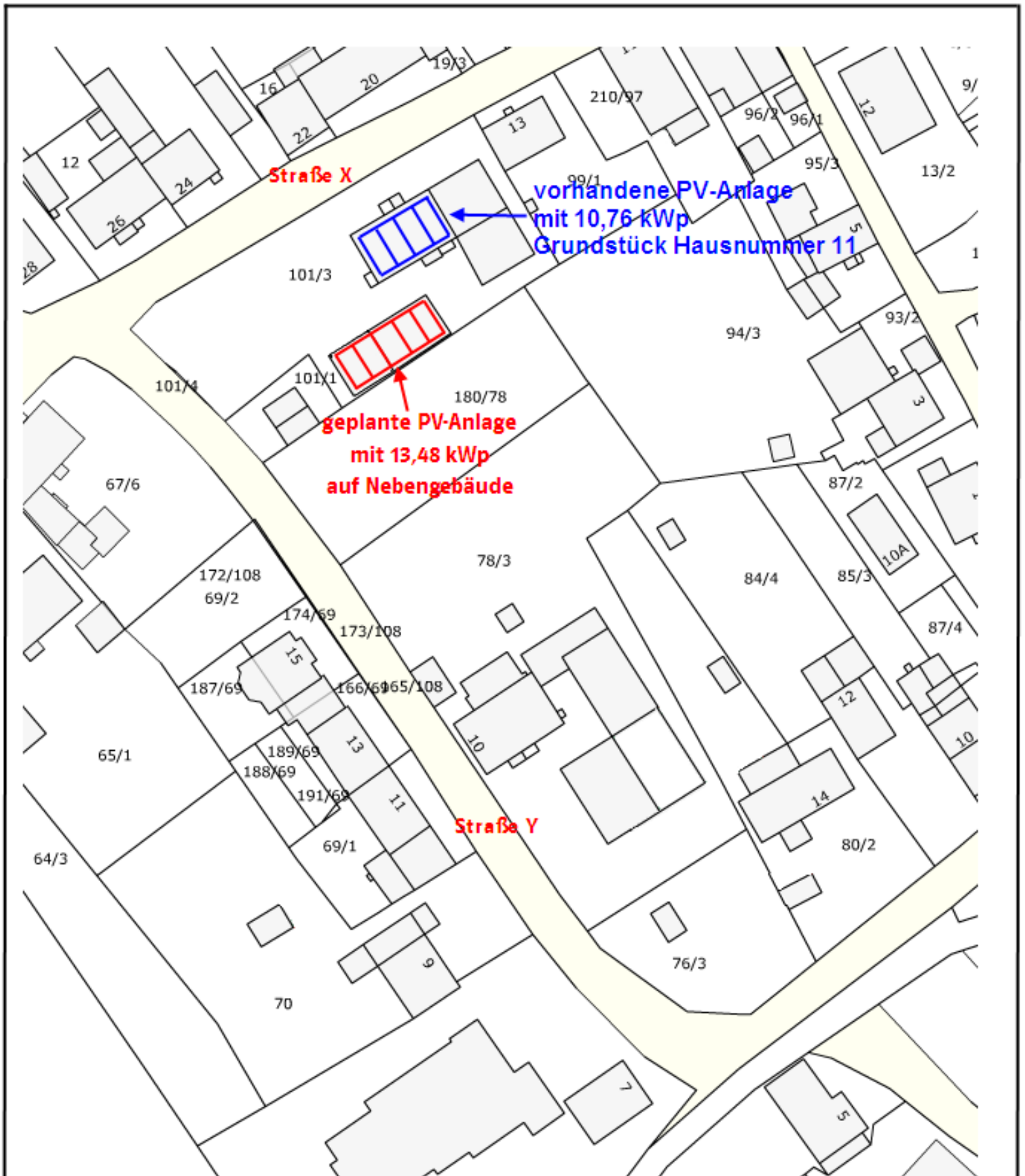
geplante Photovoltaikanlage Mustermann, Straße X, PLZ Ort
