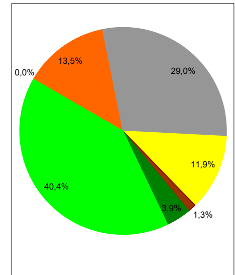
Stromerzeugung 2019 in Deutschland - Durchschnittswerte zum Vergleich
